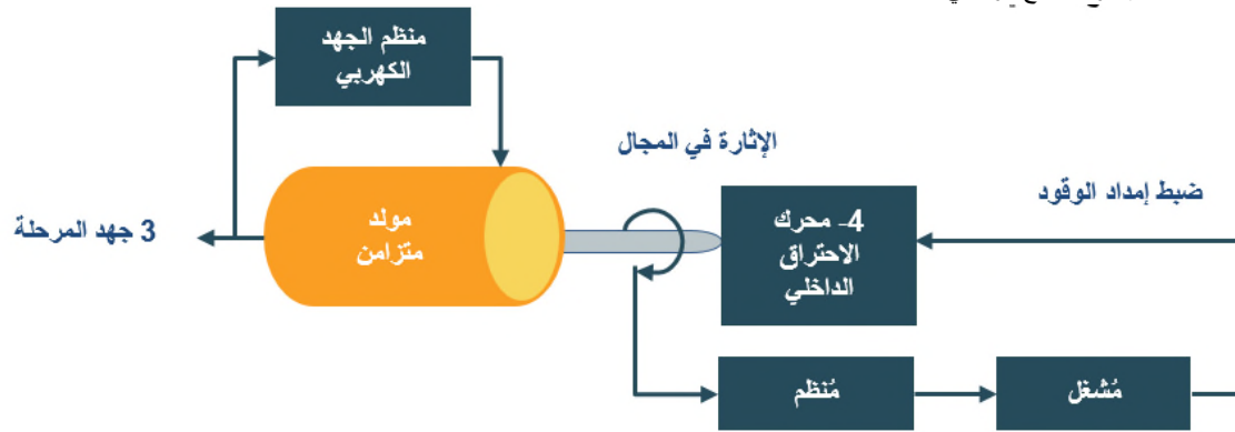
الشكل 2: أجزاء مولد الديزل
